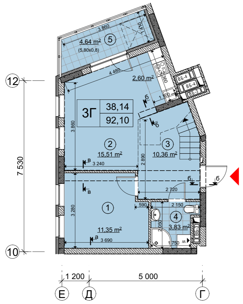
План квартири на 1-му рівні
