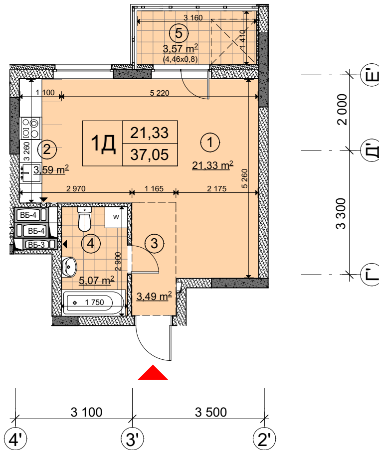
Експлікація приміщень
