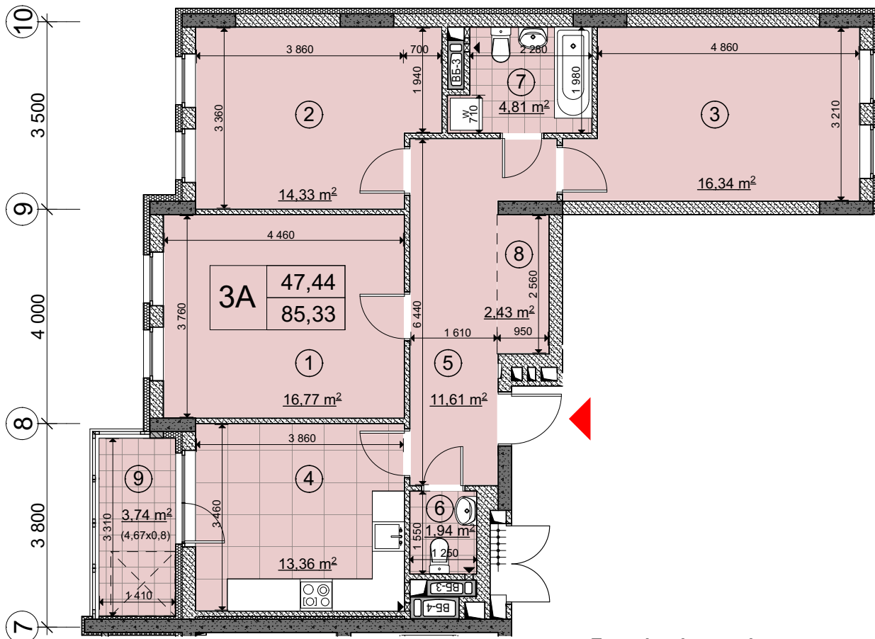
Схема розташування квартири в секції Г*
