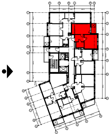
Схема розташування квартири в секції Д
