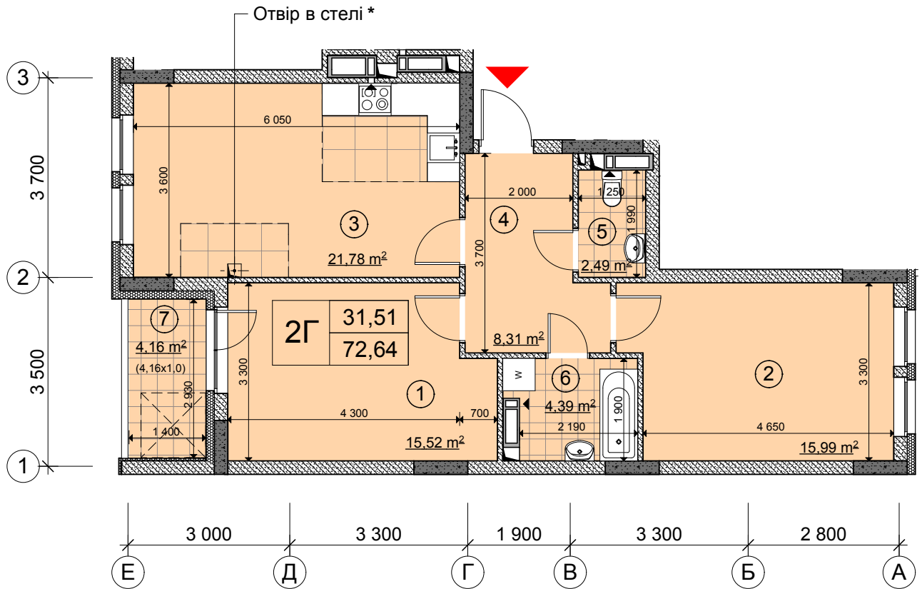
Схема розташування квартири в секції А
