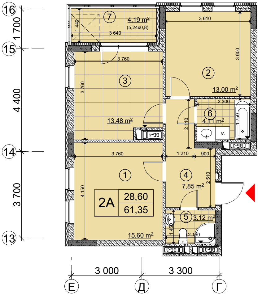
Схема розташування квартири в секції А
