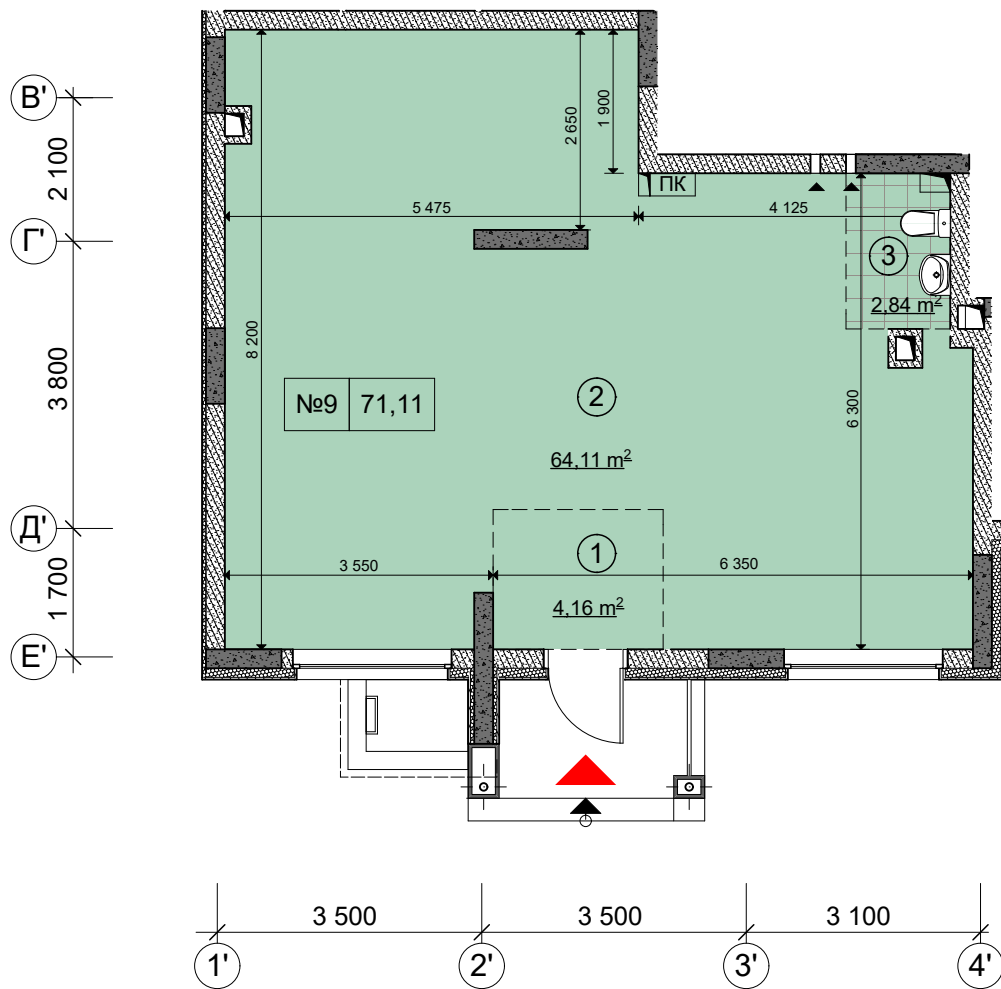
Схема розташування нежитлового приміщення в секції Д
