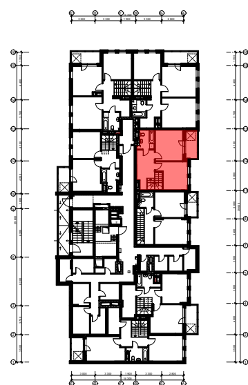
Схема розташування квартири в секції А на 17-му поверсі
