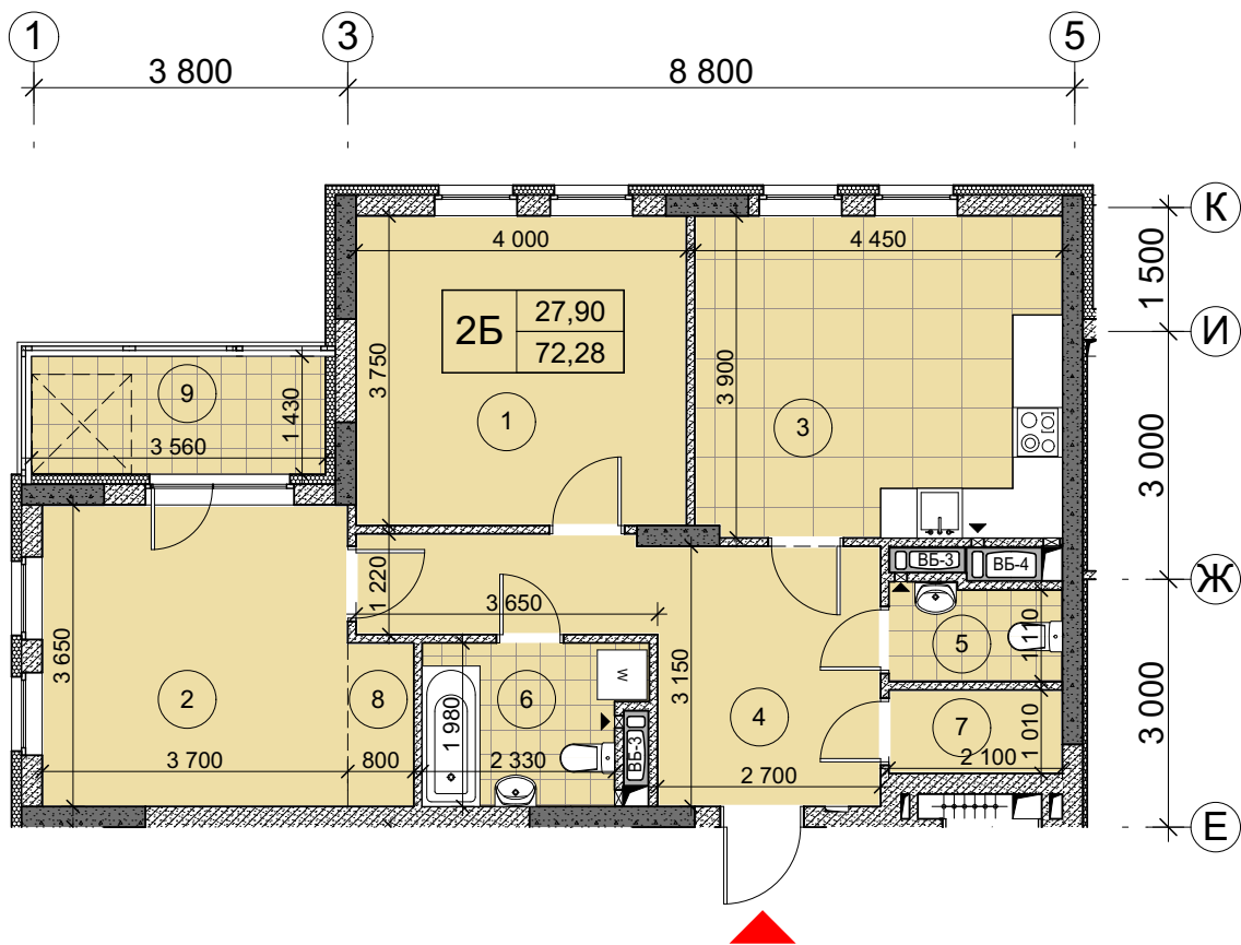
Схема розташування квартири в секції Г
