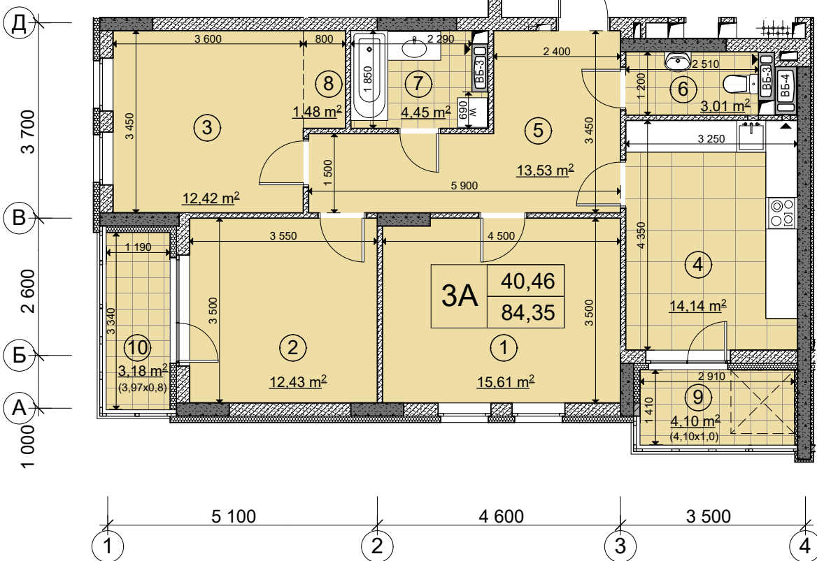
Схема розташування квартири в секції В
