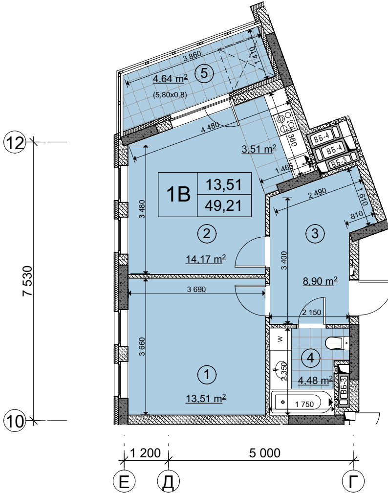
Схема розташування квартири в секції Б
