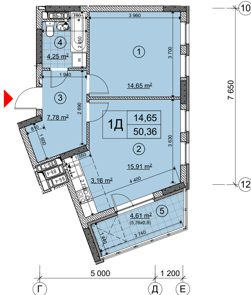
Схема розташування квартири в секції Д
