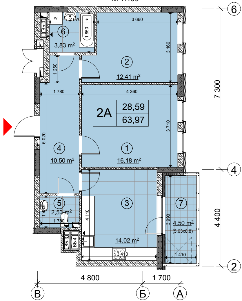
Схема розташування квартири в секції Е1
