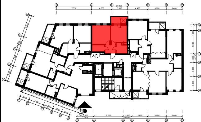
Схема розташування квартири в секції І
