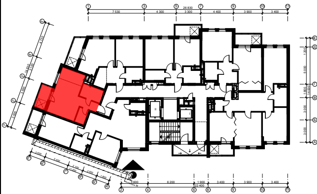
Схема розташування квартири в секції И
